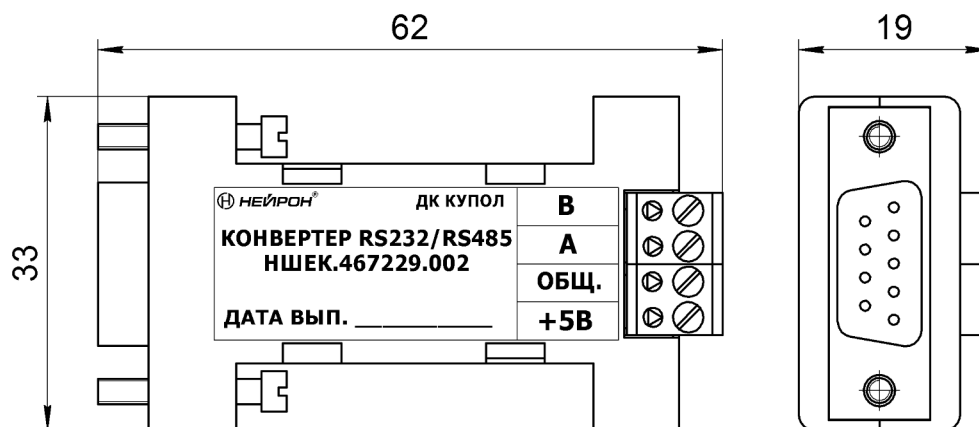
Рис.1 Внешний вид Конвертер RS232/RS485 НШЕК.467229.002
